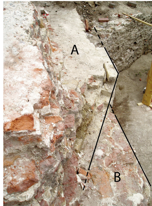
Afb. 1. Tweede stadsmuur met de oudste fase van de muur in Vlaams verband (A) en de latere aansluitende muur (B). (Foto: BAM)
