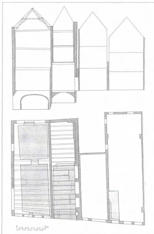
afb. 3 Brede Haven 1-2, 3, 4 en 5. Dwarsdoorsnede en platte- grondtekening. In een grijze arcering zijn de kelders weergegeven. (Tekening K. Bujdosó BAD)
